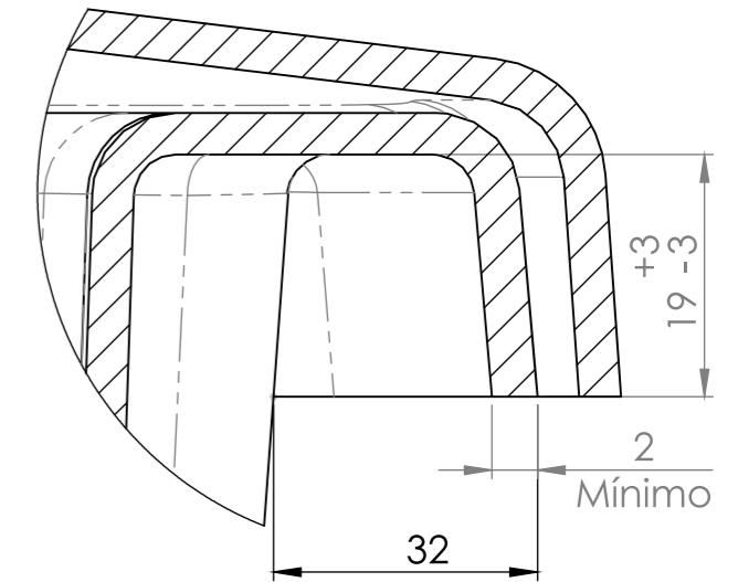
DETALHE B
