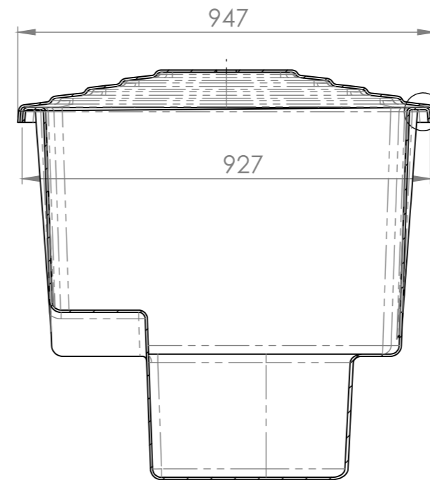
SEÇÃO A-A
