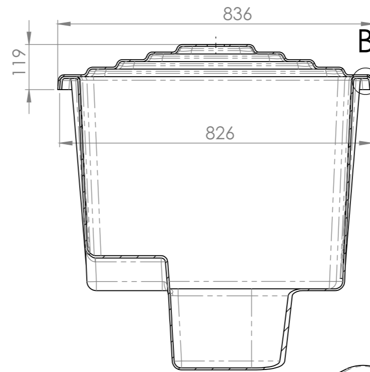
SEÇÃO A-A
