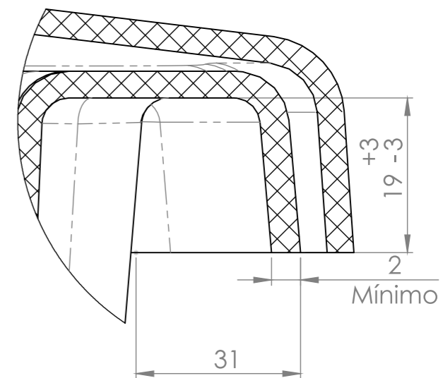
DETALHE B
